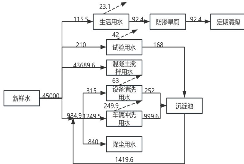
图 2-1 项目水平衡图
